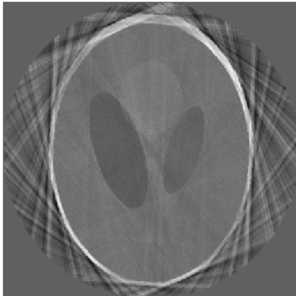
Rétroprojection filtrée avec 60 angles irréguliers
